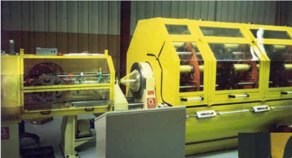
Kevlar Armieranlage Kevlar armouring line Ligne d'armage Kevlar Línea de armar Kevlar Линия армирования для Кевлара 芳纶纱铠装机
