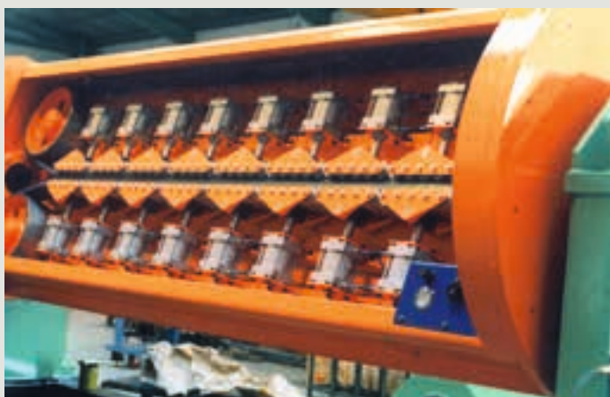
Rotierender Bandabzug Rotating belt-type capstan Chenille rotative Oruga giratoria Вращающаяся ленточная тяга 旋转履带牵引机
