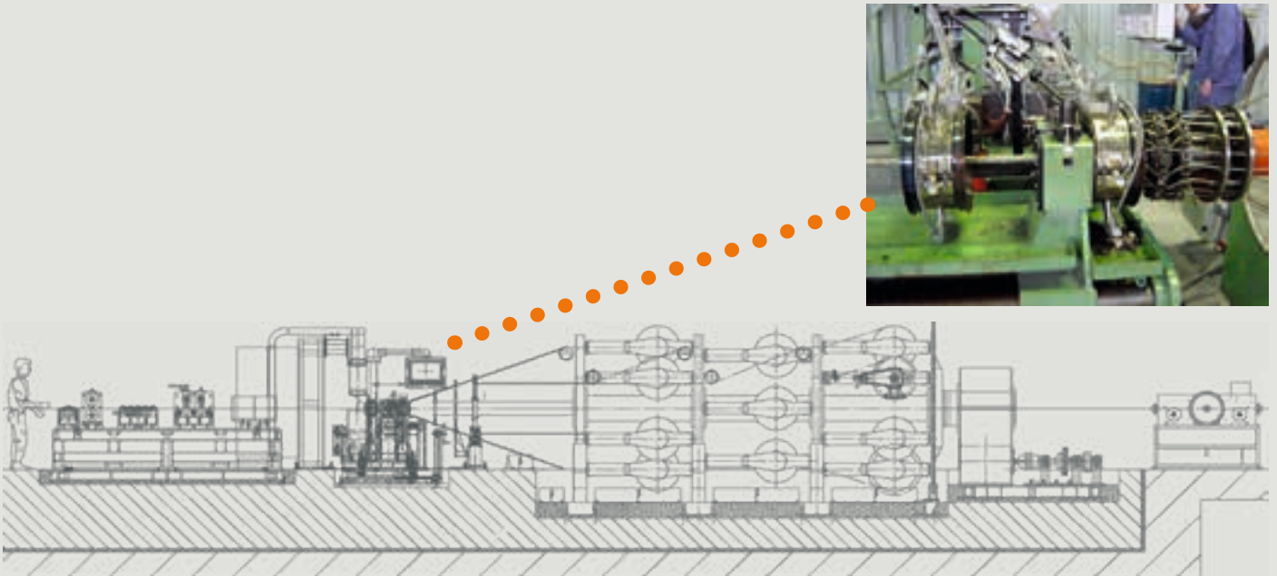
Extruder für PP Einspritzung in Kernseil Extruder for PP injection into rope core Extrudeuse pour injection de PP dans le centre du toron métallique Extrusora para inyección de PP dentro del núcleo de cable de acero Экструдер для впрыска полипропилена в сердечник каната PP料注芯机
