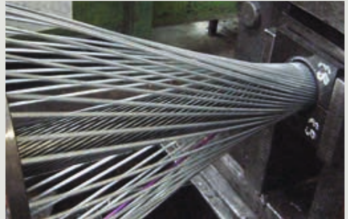
Verseilung von Stahldrähten Stranding of steel wires Assemblage des fils d'acier Cableado de alambres de acero Скрутка стальных проволок 用于绞合钢丝
